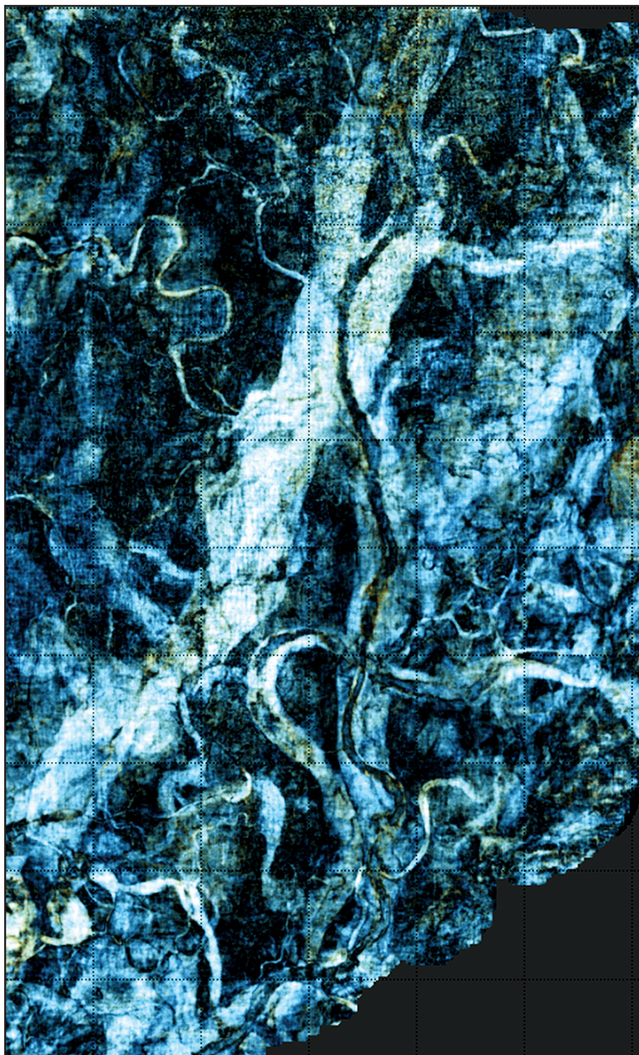
Рисунок 2 – Погоризонтный срез куба цветовой суммы кубов спектральной декомпозиции HDFD (ffA GeoTerGic)
