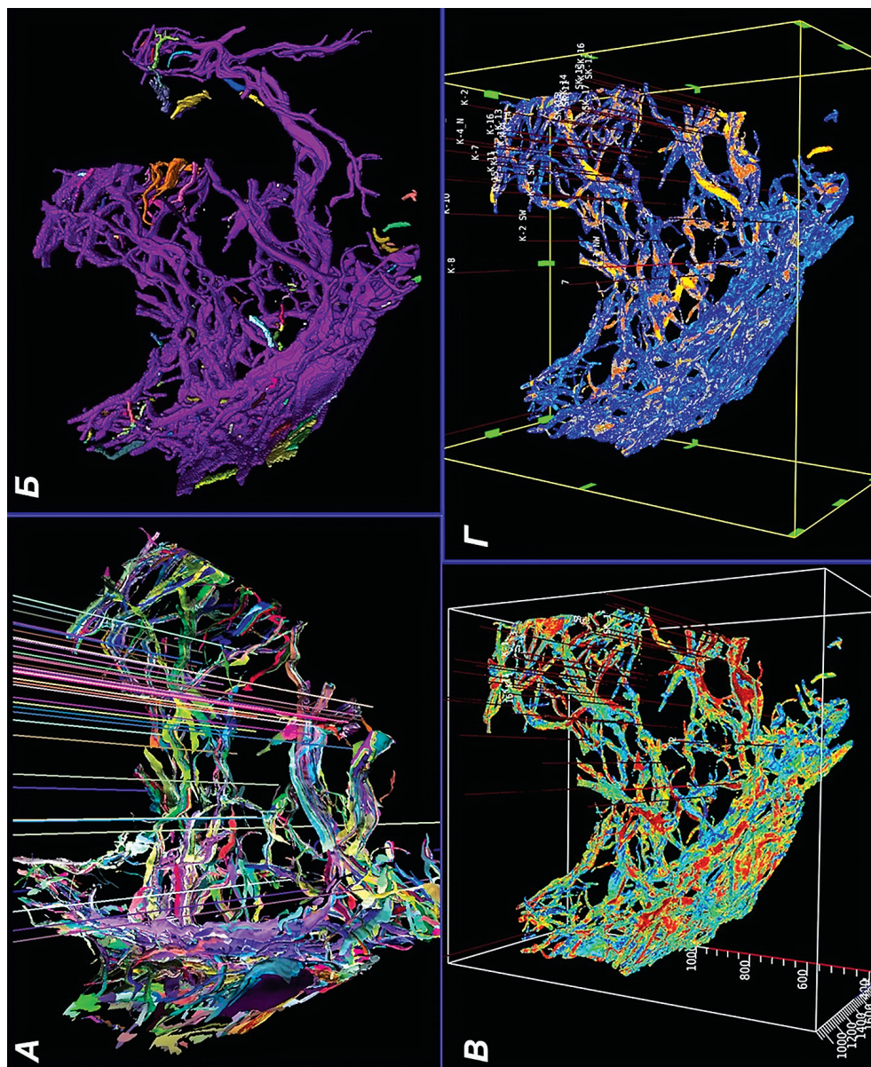
Рисунок 7 – Выделенные геологические тела палеорусел Eilis PaleoScan (А), Petrel (Б), геологические тела палеорусел, заполненные данными куба сейсмических фаций Halliburton GeoProbe (В), и куба атрибута Sweetness (Г)
