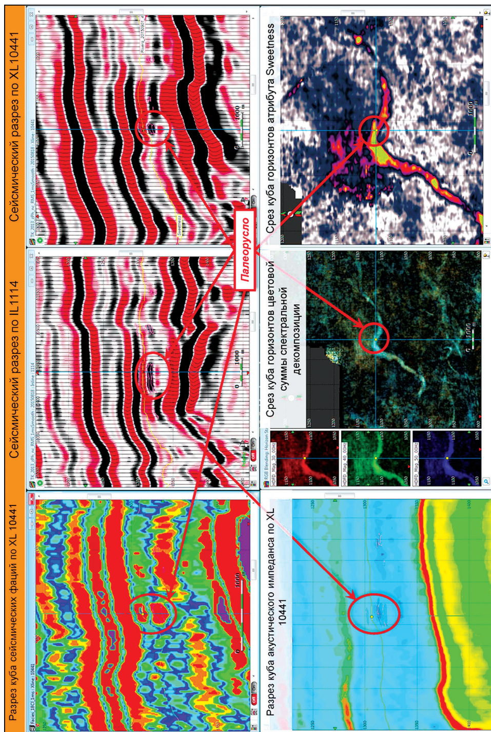
Рисунок 8 – Прослеживание геологических тел палеорусел по кубам горизонтов сейсмических атрибутов, фаций, спектральной декомпозиции и акустического импеданса (Eiis PaleoScan)
